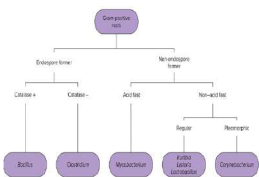
Gambar 8.8: Outline pemisahan untuk batang Gram-positif
