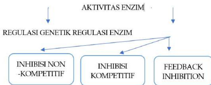
Gambar 6.2:. Regulasi Aktivitas Enzim
